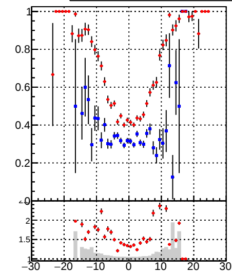
Fake rate vs \sqrt{s} DQM_CKF DQM_BDT_CKF
