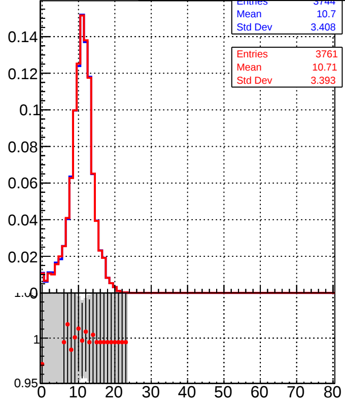
DQM_CKF DQM_BDT_CKF
