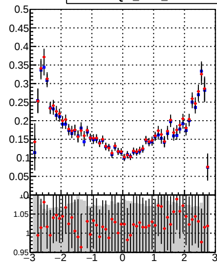
■ DQM_CKF ■ DQM_BDT_CKF
