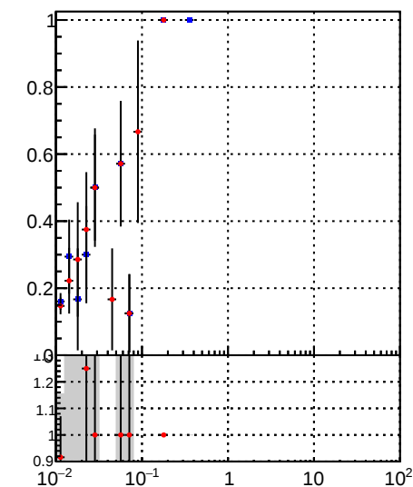
Fake rate vs v_z DQM_CKF DQM_BDT_CKF
