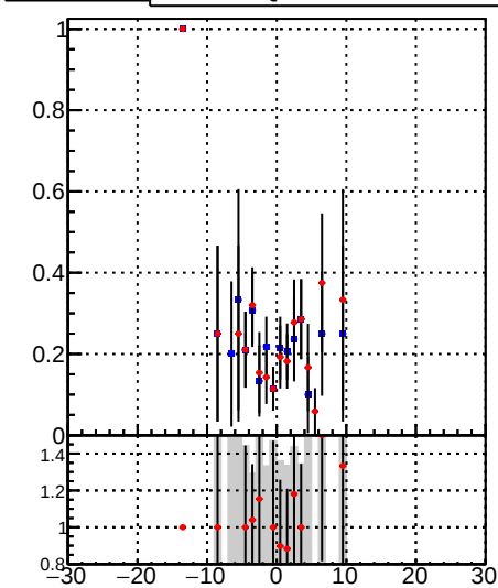
Fake rate vs v_z DQM_CKF DQM_BDT_CKF
