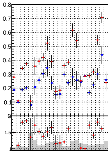
Fake rate vs. — DQM CKF — DQM BDT CKF
