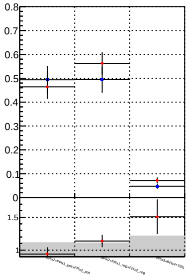
Fake rate vs. — DQM_CKF — DQM_BDT_CKF
