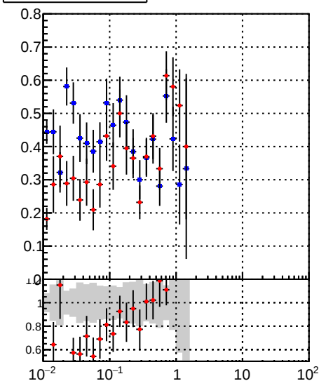
■ DQM_CKF ● DQM_BDT_CKF
