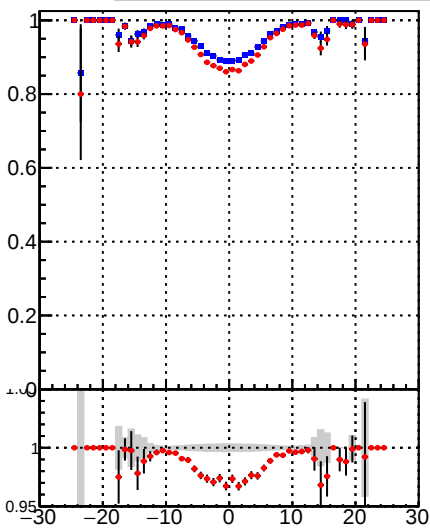
DQM_CKF DQM_BDT_CKF Fake rate vs v
