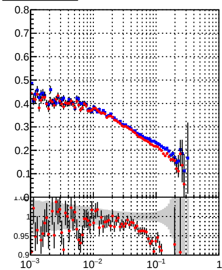
■ DQM_CKF ● DQM_BDT_CKF
