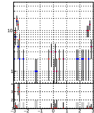
—•— DQM_CKF —+— DQM_BDT_CKF
