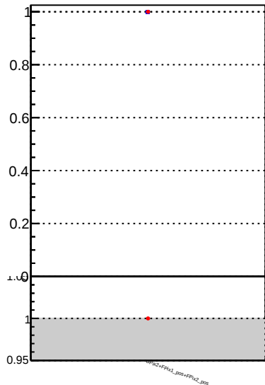
Fake rate vs. DQM_CKF DQM_BDT_CKF
