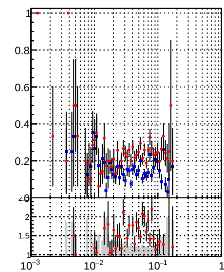
Fake rate vs \sqrt{s} DQM_CKF DQM_BDT_CKF
