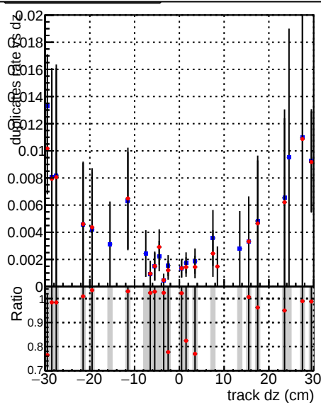
al__mkFitbase1__RECO al__mkFitbase2__RECO
