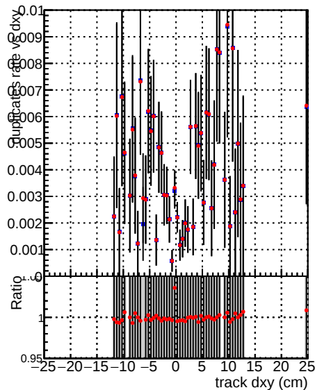
al__mkFitbase1__RECO al__mkFitbase2__RECO
