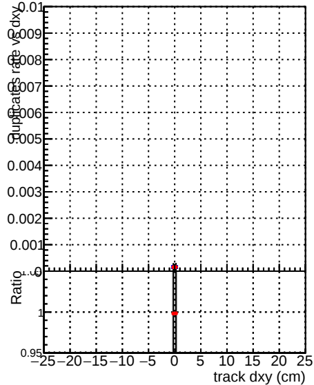
al__mkFitbase1__RECO al__mkFitbase2__RECO
