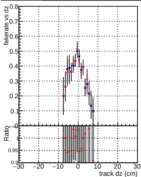
█ █ DQM V0001_R0000000001 Global mkFitbase1 RECO █ █ DQM V0001_R0000000001 Global mkFitbase2 RECO
