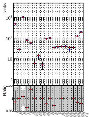
Legend: - Global mkFitbase1 RECO - Global mkFitbase2 RECO
