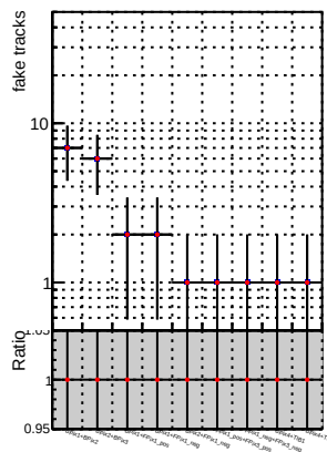
Legend: - Global mkFitbase1 RECO - Global mkFitbase2 RECO
