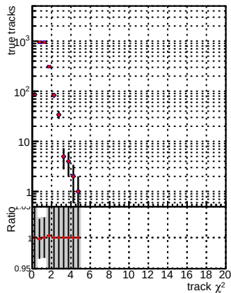
Legend: - Global mkFitbase1 RECO - Global mkFitbase2 RECO
