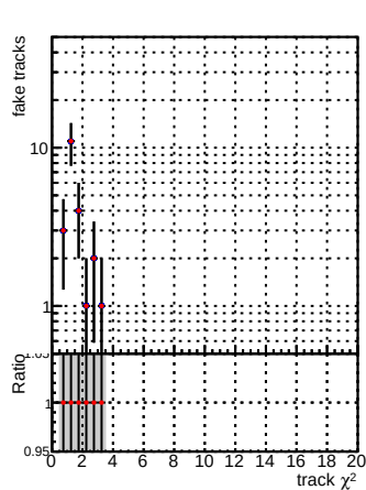
Legend: - Global mkFitbase1 RECO - Global mkFitbase2 RECO
