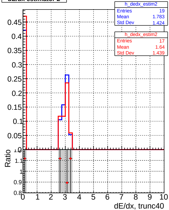
dE/dx estimator 2
