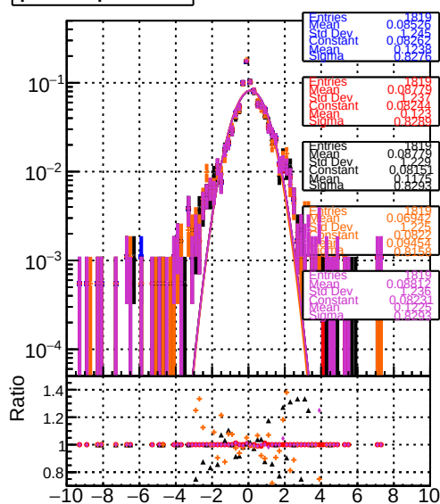
pull of \theta parameter 0.20 eta2p5to4p0
