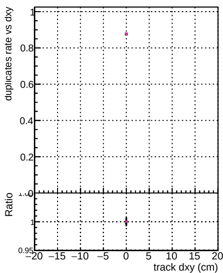
eta2p0to2p5
