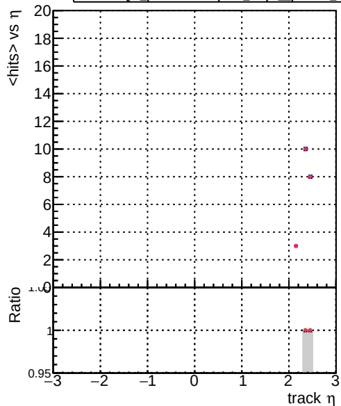
DOM original step2 pt1to20 eta2p0to2p5 DOM mkrfit_step2 pt1to20 eta2p0to2p5 DOM angle_step2 pt1to20 eta2p0to2p5 DOM fast_step2 pt1to20 eta2p0to2p5 DOM pixelCPEtemplate_step2 pt1to20 eta2p0to2p5
