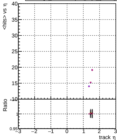
DOM original_step2_pt1to20_eta1p4to1p6 DOM mkrfit_step2_pt1to20_eta1p4to1p6 DOM angle_step2_pt1to20_eta1p4to1p6 DOM fast_step2_pt1to20_eta1p4to1p6 DOM pixelCPEtemplate_step2_pt1to20_eta1p4to1p6
