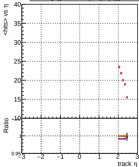
DOM original step2 pTto1000 eta2p0to2p5 DOM mkrfit step2 pTto1000 eta2p0to2p5 DOM angle step2 pTto1000 eta2p0to2p5 DOM fast step2 pTto1000 eta2p0to2p5 DOM pixelCPE template step2 pTto1000 eta2p0to2p5
