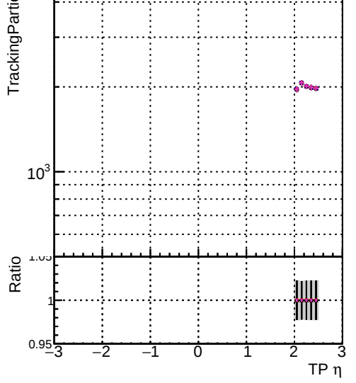
N of simulated tracks vs eta
