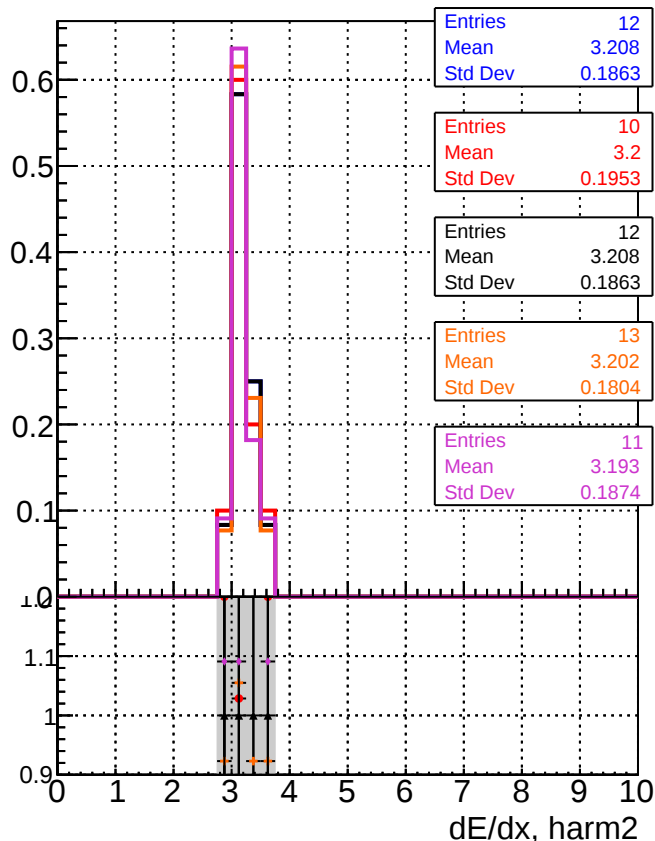
dE/dx estimator 1
