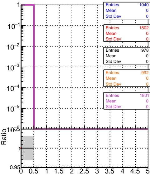
mean hit <math>\langle \text{hits} \rangle \text{ vs } \eta</math>
