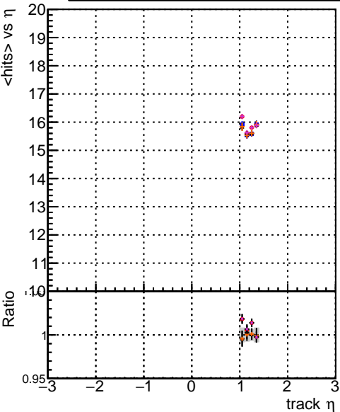
mean hit <math>\langle \text{hits} \rangle \text{ vs } \eta</math>
