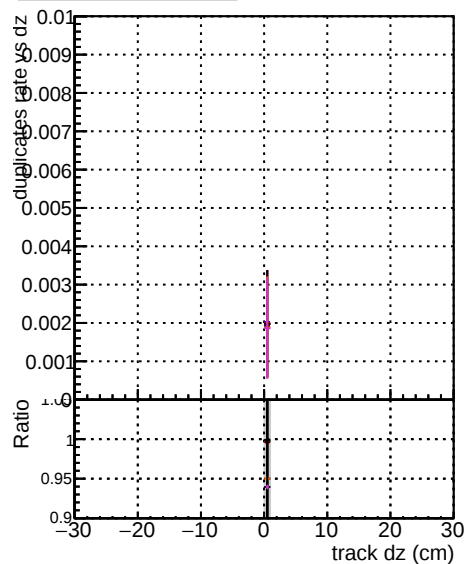
ttbar-phase1-newgeom
