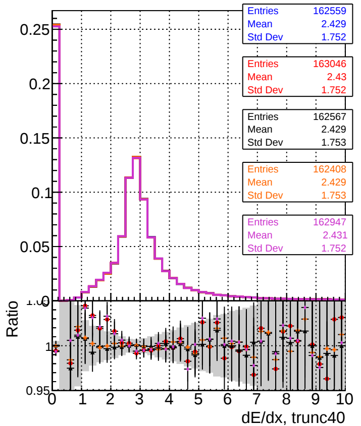
dE/dx estimator 2
