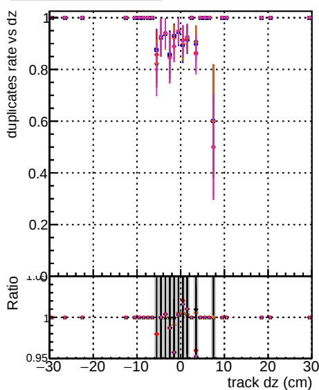
pt1to20 eta2p0to2p5
