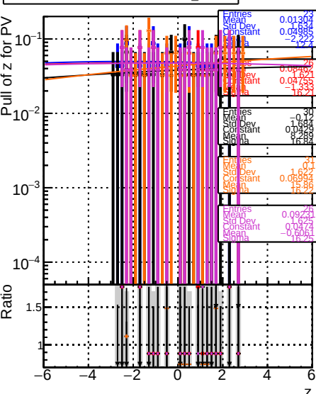
RecoPVAssoc2GenPVMatched_PullZ
