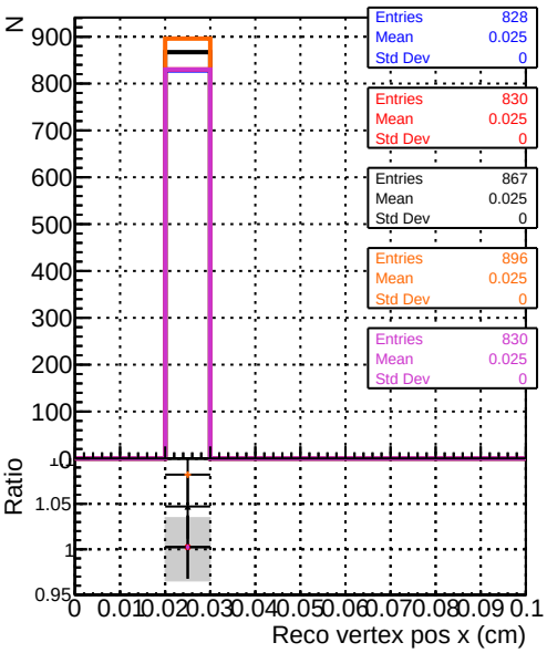
Recons DOM original step2 pt1to20 eta1p6to2p0 DOM mkrFit_step2 pt1to20 eta1p6to2p0 DOM angle_step2 pt1to20 eta1p6to2p0 DOM fast_step2 pt1to20 eta1p6to2p0 DOM pixelCPEGeneric_step2 pt1to20 eta1p6to2p0
