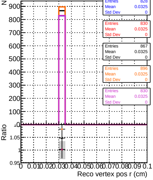
Recons DOM original step2 pt1to20 eta1p6to2p0 DOM mkrFit_step2 pt1to20 eta1p6to2p0 DOM angle_step2 pt1to20 eta1p6to2p0 DOM fast_step2 pt1to20 eta1p6to2p0 DOM pixelCPEGeneric_step2 pt1to20 eta1p6to2p0
