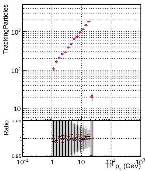
—•— DQM original step2 pt1to20 eta1p4to1p6 —•— DQM mkFit step2 pt1to20 eta1p4to1p6 —•— DQM angle step2 pt1to20 eta1p4to1p6 —•— DQM fast step2 pt1to20 eta1p4to1p6 —•— DQM pixelCPEGeneric step2 pt1to20 eta1p4to1p6
