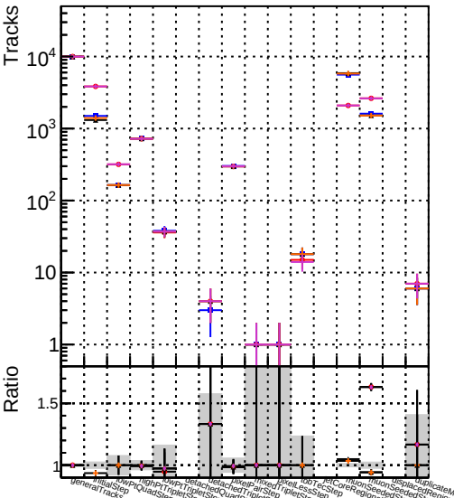
Number Legend DOM original step2 ptlto20 eta1p4to1p6 ● DOM original step2 ptlto20 eta1p4to1p6 ○ mkf1st step2 ptlto20 eta1p4to1p6 △ angle step2 ptlto20 eta1p4to1p6 + fast step2 ptlto20 eta1p4to1p6 * DOM pixelCPEGeneric step2 ptlto20 eta1p4to1p6
