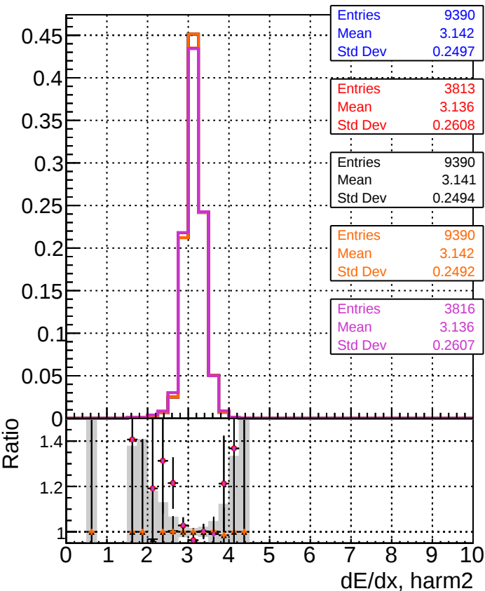
— DQM original step2 pt1to20 eta1p4to1p6 — DQM mkFit step2 pt1to20 eta1p4to1p6 — DQM angle step2 pt1to20 eta1p4to1p6 — DQM fast step2 pt1to20 eta1p4to1p6 — DQM pixelCPEGeneric step2 pt1to20 eta1p4to1p6
