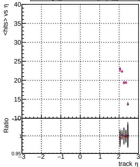
DOM original step2 pTto1000 eta2p0to2p5 DOM mkrfit step2 pTto1000 eta2p0to2p5 DOM angle step2 pTto1000 eta2p0to2p5 DOM fast step2 pTto1000 eta2p0to2p5 DOM pixelCPEGeneric step2 pTto1000 eta2p0to2p5
