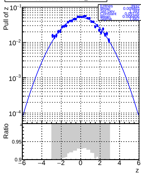
RecoAllAssoc2GenMatched_PullZ
