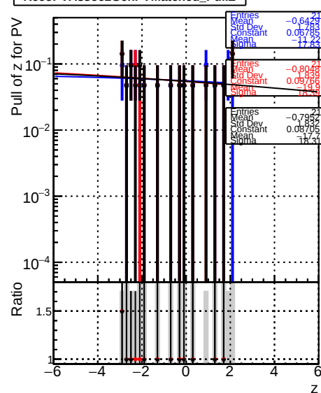
RecoPVAssoc2GenPVMatched_PullZ
