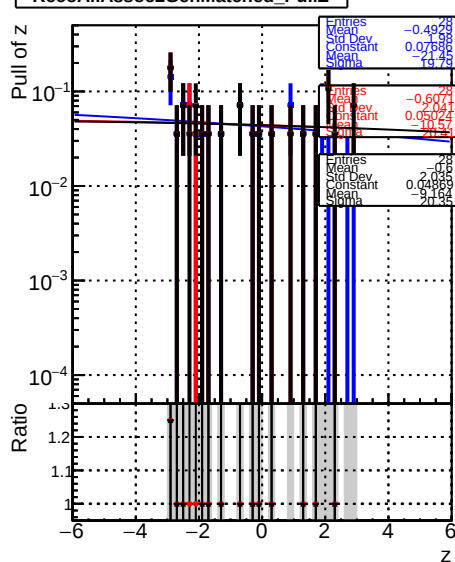
RecoAllAssoc2GenMatched_PullZ
