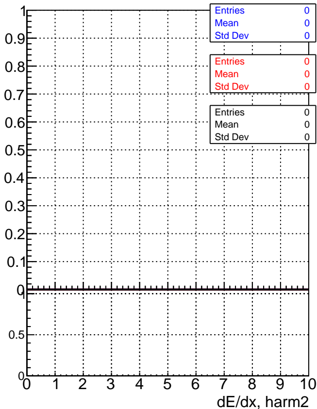
dE/dx estimator 1
