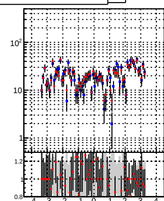
pT eta
