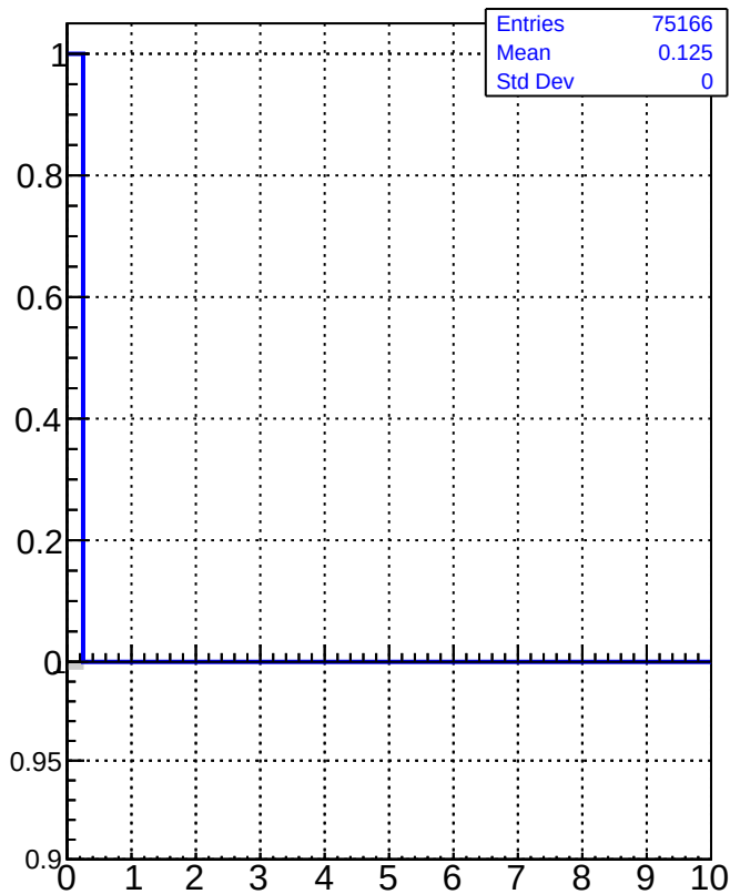
dE/dx estimator 1
