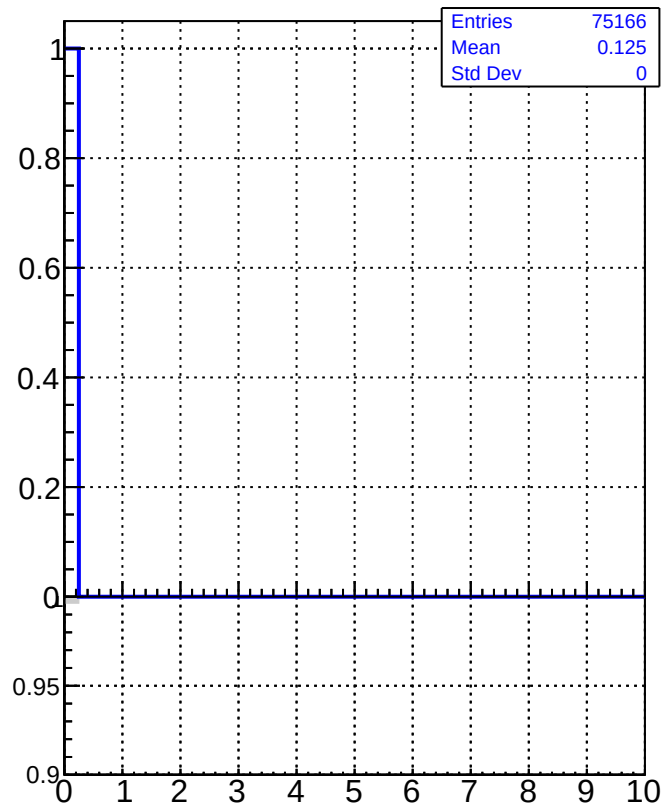
dE/dx estimator 2
